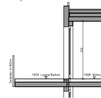
Prinzipschnitt:
